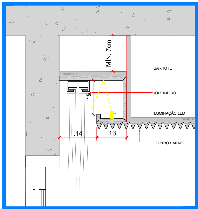
DET. 03 - CORTINEIRO ILUMINADO 1:10
