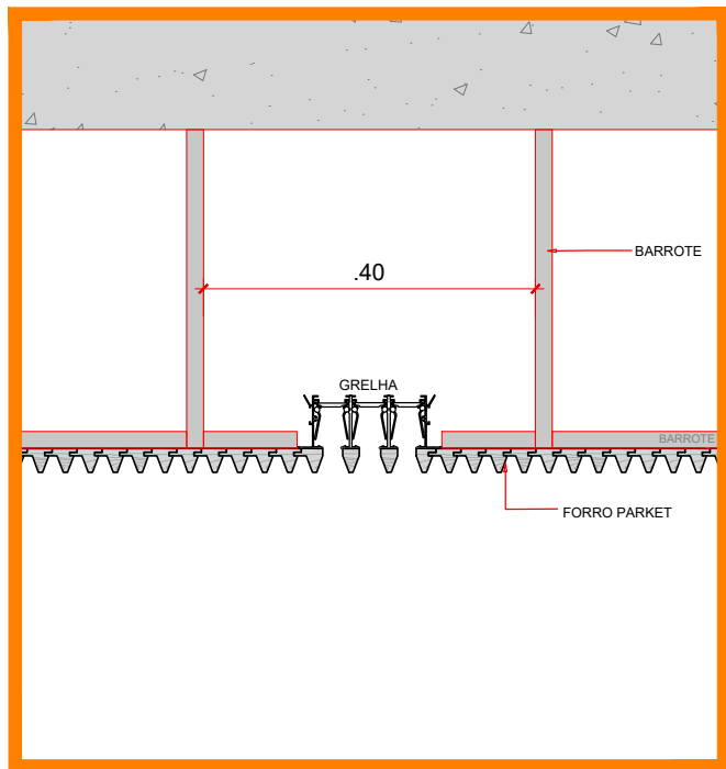
DET. 01 - GRELHA 1:10
